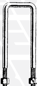
26 - 722678 ø 16x60x130 27 - 722735 ø 16x60x140 28 - 722679 ø 16x60x150 29 - 722744 ø 16x60x160 30 - 722685 ø 16x60x180 31 - 722686 ø 16x60x200
