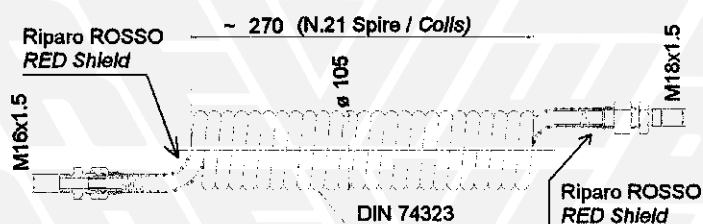
14 - 711808 NERO con RIPARI ROSSI/BLACK with RED SHIELDS
