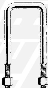
16 - 722020 \varnothing 16x70x250 17 - 722021 \varnothing 16x70x270 18 - 722574 \varnothing 16x70x280 19 - 722022 \varnothing 16x70x300 20 - 722576 \varnothing 16x70x330 21 - 722577 \varnothing 16x70x350 22 - 722578 \varnothing 16x70x370
