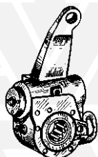
10 - 727639 Dx / RH 11 - 727640 Sx / LH
