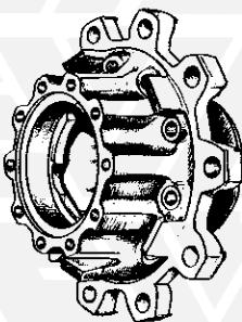
18 - 713774 nudo / bare 19 - 713798 completo / assembly
