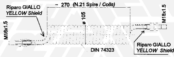
15 - 711809 NERO con RIPARI GIALLI/BLACK with YELLOW SHIELDS
