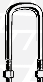
22 - 722129 \varnothing 22x93x197 23 - 722130 \varnothing 22x93x240
