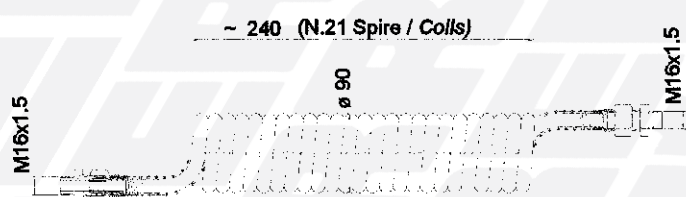
7 - 711800 ROSSO/RED 8 - 711801 BLU/BLUE 9 - 711802 GIALLO/YELLOW
