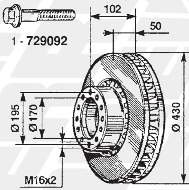
2 - 713456 con bulloni / c/w bolts
