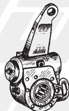
17 - 727639 Dx / RH 18 - 727640 Sx / LH
