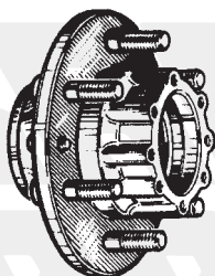
22 - 713526 c/colonnette / c/w studs
