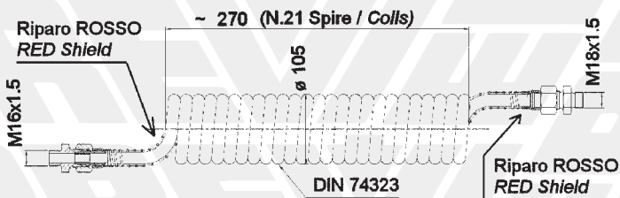
~ 270 (N.21 Spire / Colls) 14 - 711808 NERO con RIPARI ROSSI/BLACK with RED SHIELDS DIN 74323
