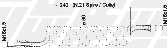
~ 240 (N.21 Spire / Colls) 7 - 711800 ROSSO/RED 8 - 711801 BLU/BLUE 9 - 711802 GIALLO/YELLOW
