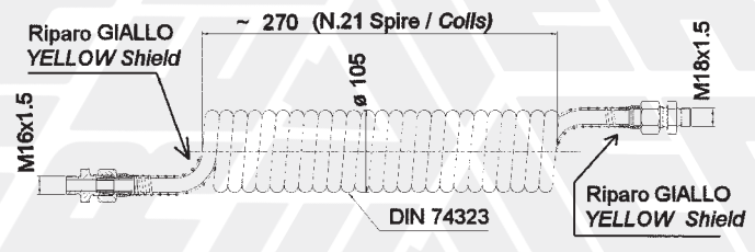
~ 270 (N.21 Spire / Colls) 15 - 711809 NERO con RIPARI GIALLI/BLACK with YELLOW SHIELDS DIN 74323
